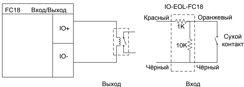
Рис. Схема подключения встроенных входов/выходов
